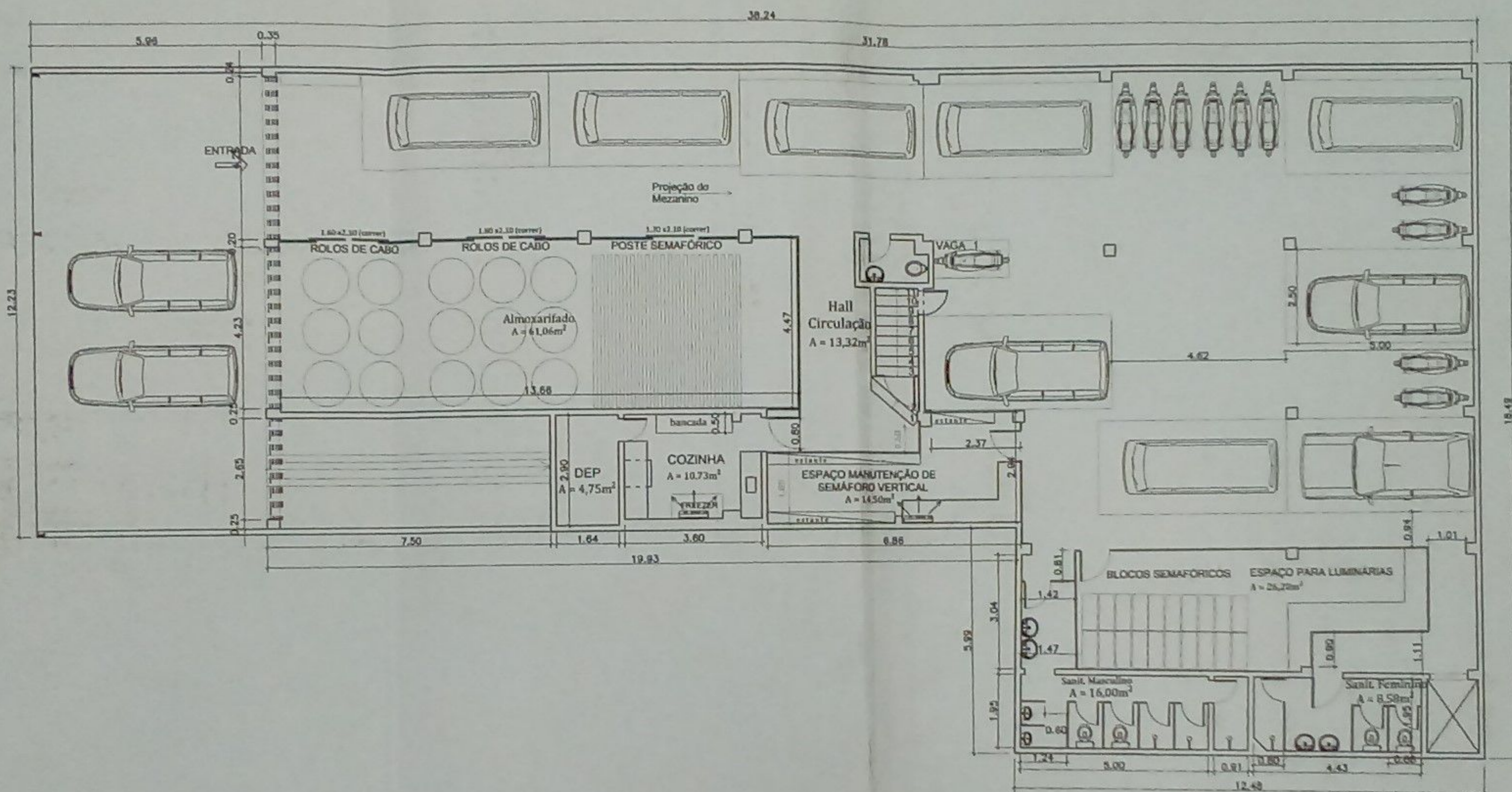
PLANTA BAIXA PAVIMENTO TÉRREO Escala 1/125
