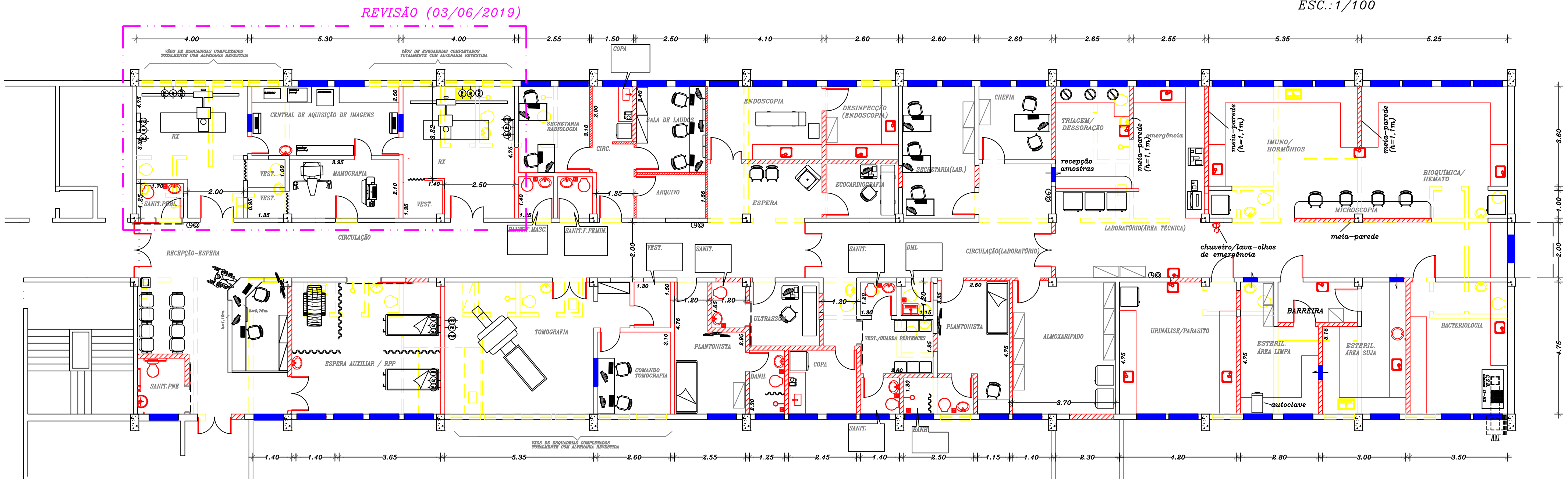
PLANTA - BAIXA/LAYOUT DEMOLIR/CONSTRUIR ESC.: 1/100
