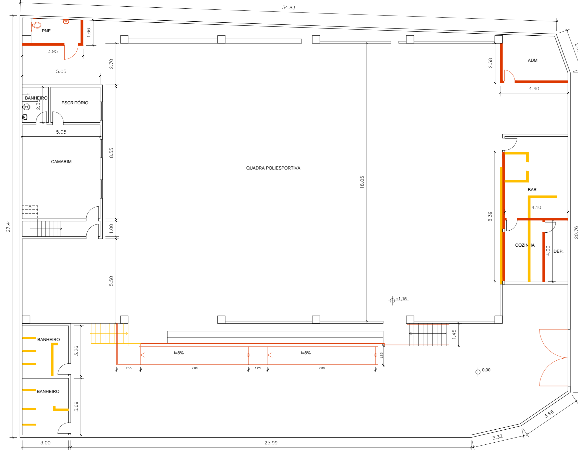
1 PLANTA DE DEMOLIR E CONSTRUIR ESCALA 1 / 125
