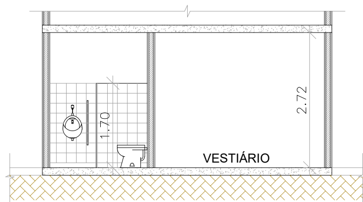
Corte AA' - Esc. 1/75
