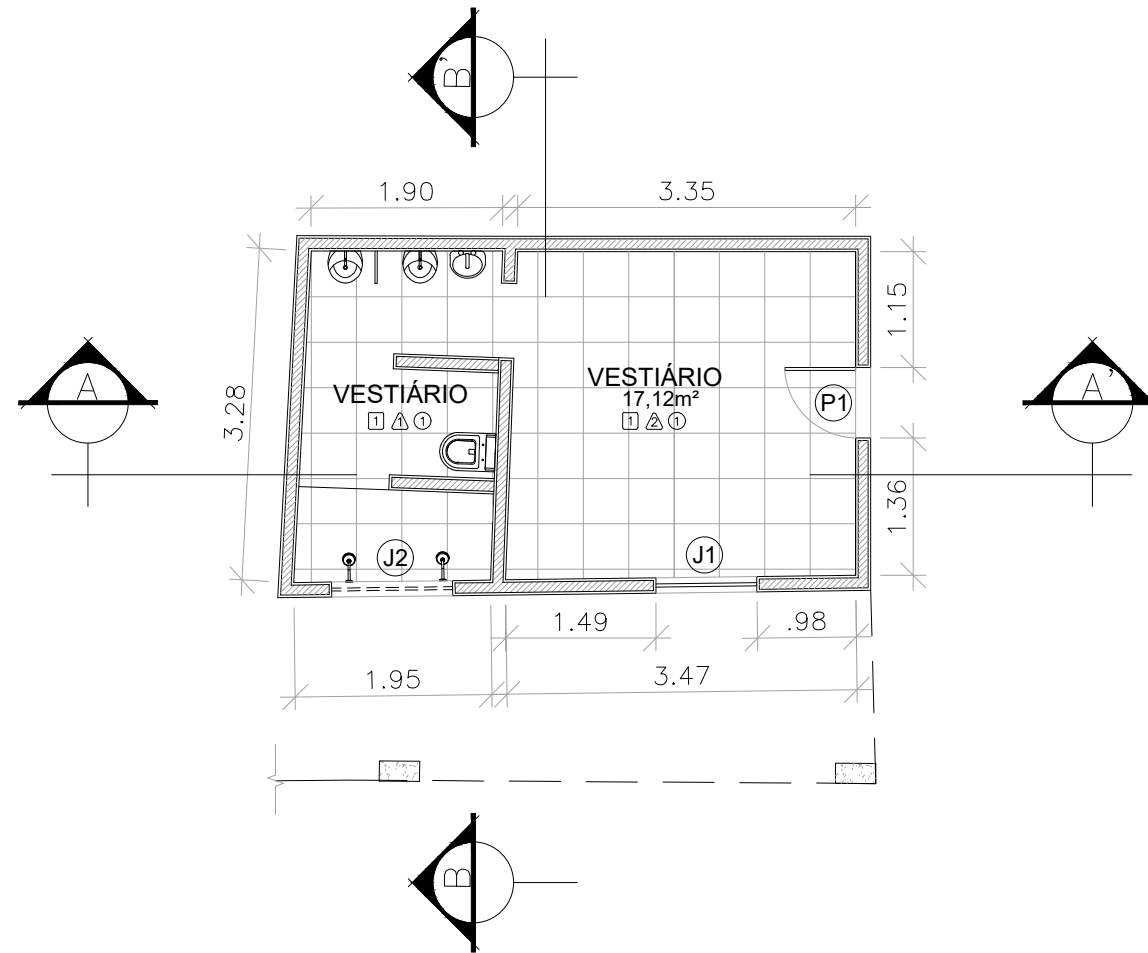
Planta Baixa - Esc. 1/75
