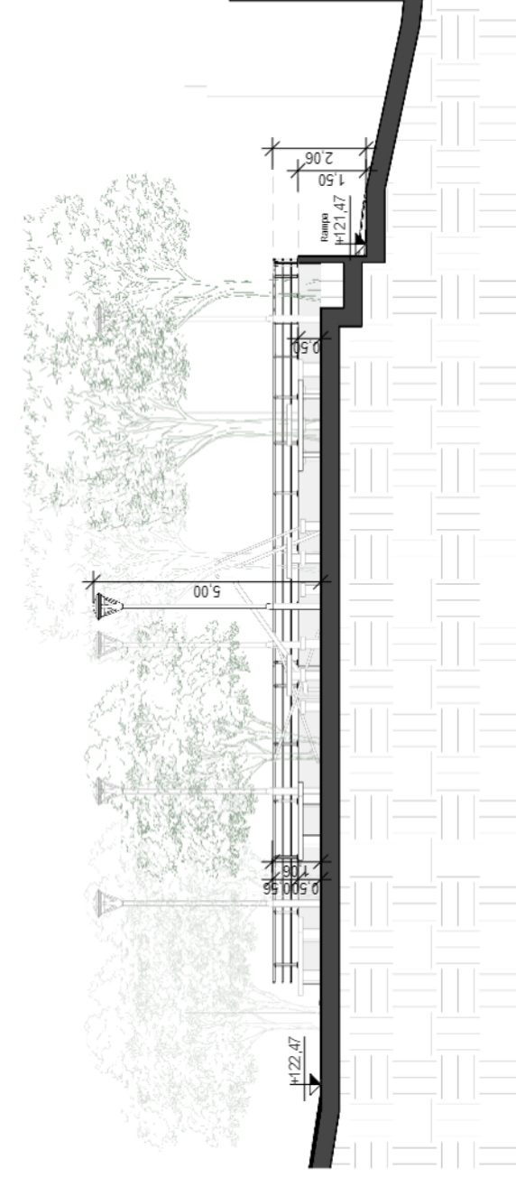
4 CORTE TRANSVERSAL
