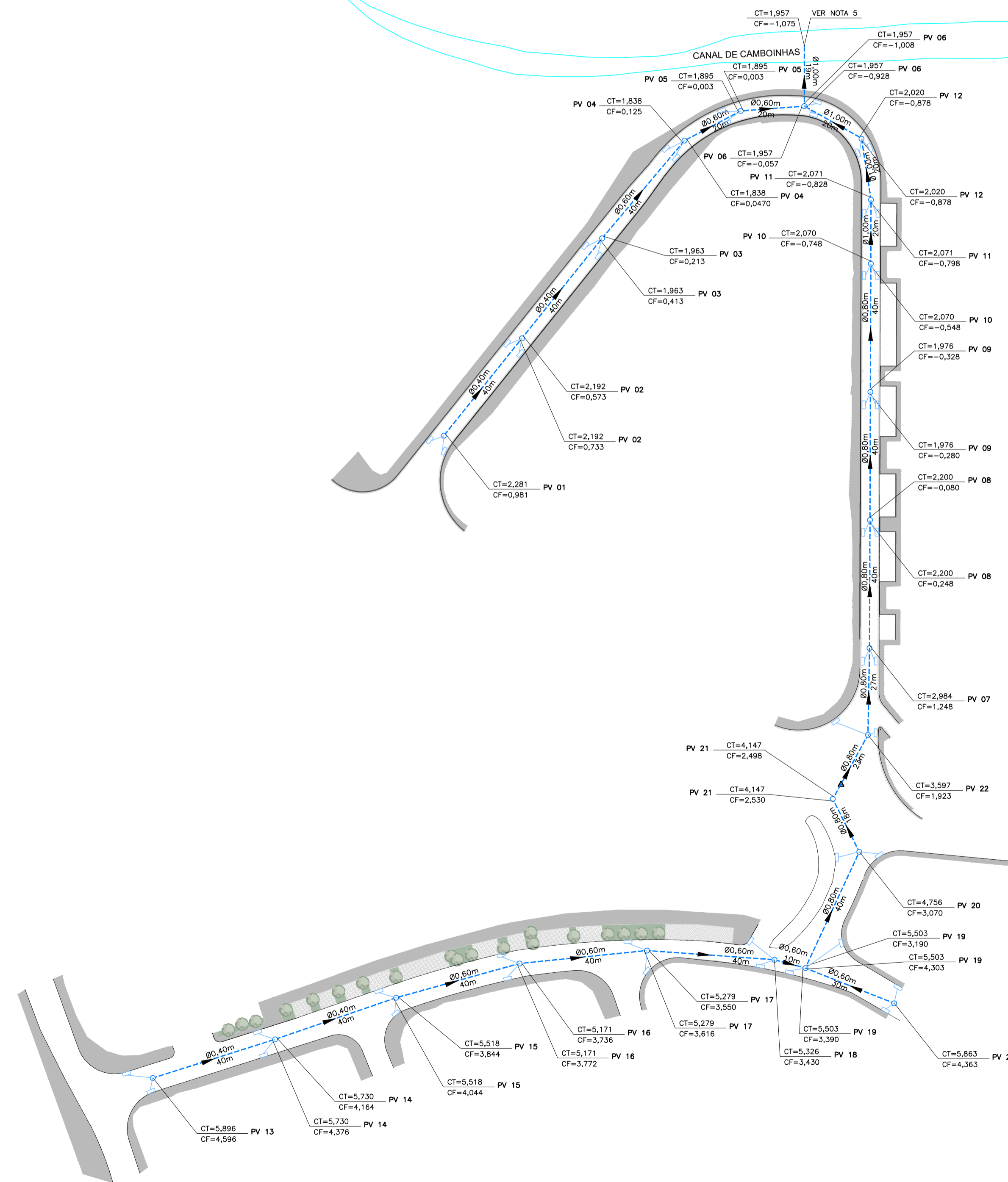
PLANTA ESCALA 1:1000
