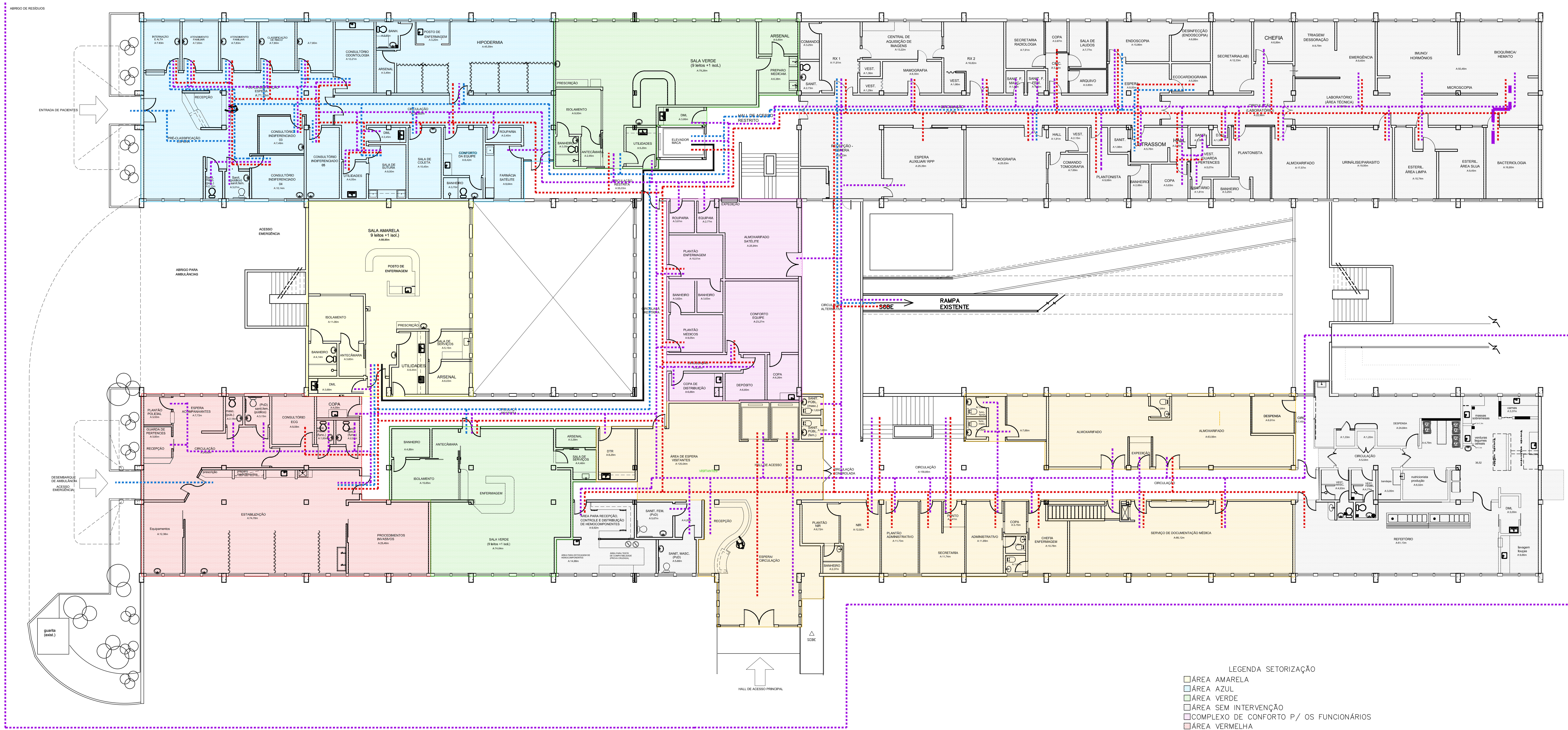
01 - HMCT - PLANTA BAIXA TÉRREO SETORIZAÇÃO E FLUXOS ESCALA - 1/100
