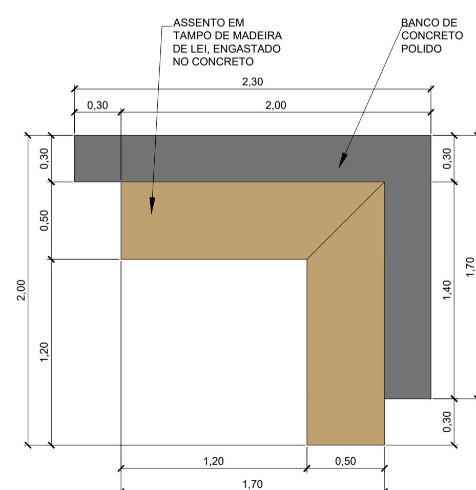
BANCO - BC 02 - Planta Baixa Esc. 1/25
