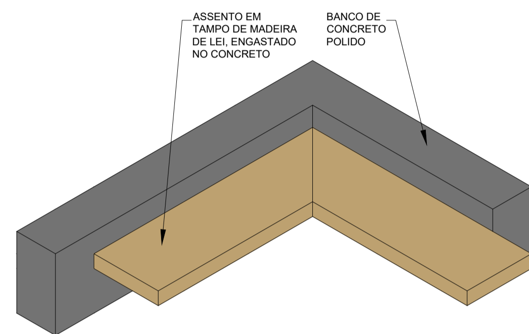
BANCO - BC 02 - Perspectiva Esc. 1/25
