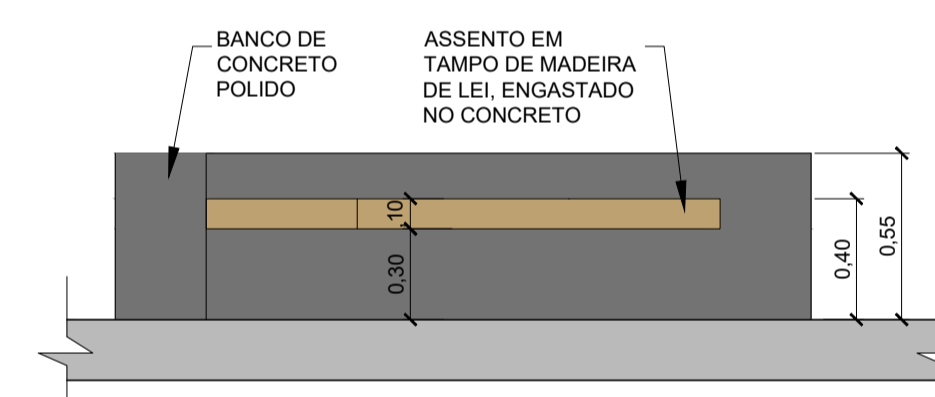
BANCO - BC 03 - Vista Frontal Esc. 1/25
