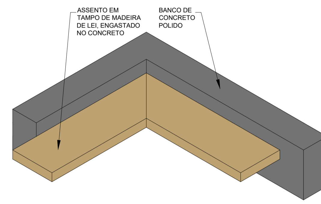
BANCO - BC 03 - Perspectiva Esc. 1/25
