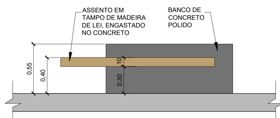
BANCO - BC 01 - Vista Frontal Esc. 1/25
