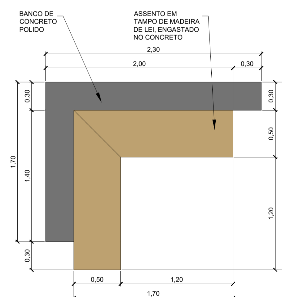
BANCO - BC 03 - Planta Baixa Esc. 1/25
