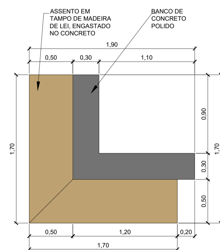
BANCO - BC 01 - Vista Frontal Esc. 1/25
