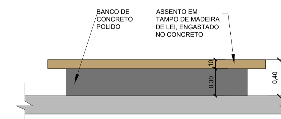
BANCO - BC 04 - Vista Frontal Esc. 1/25
