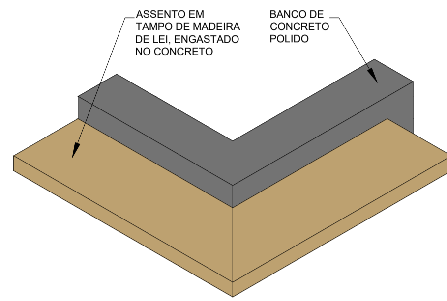
BANCO - BC 01 - Perspectiva Esc. 1/25
