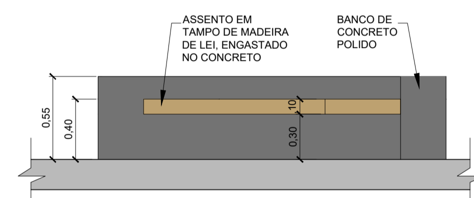
BANCO - BC 02 - Vista Frontal Esc. 1/25
