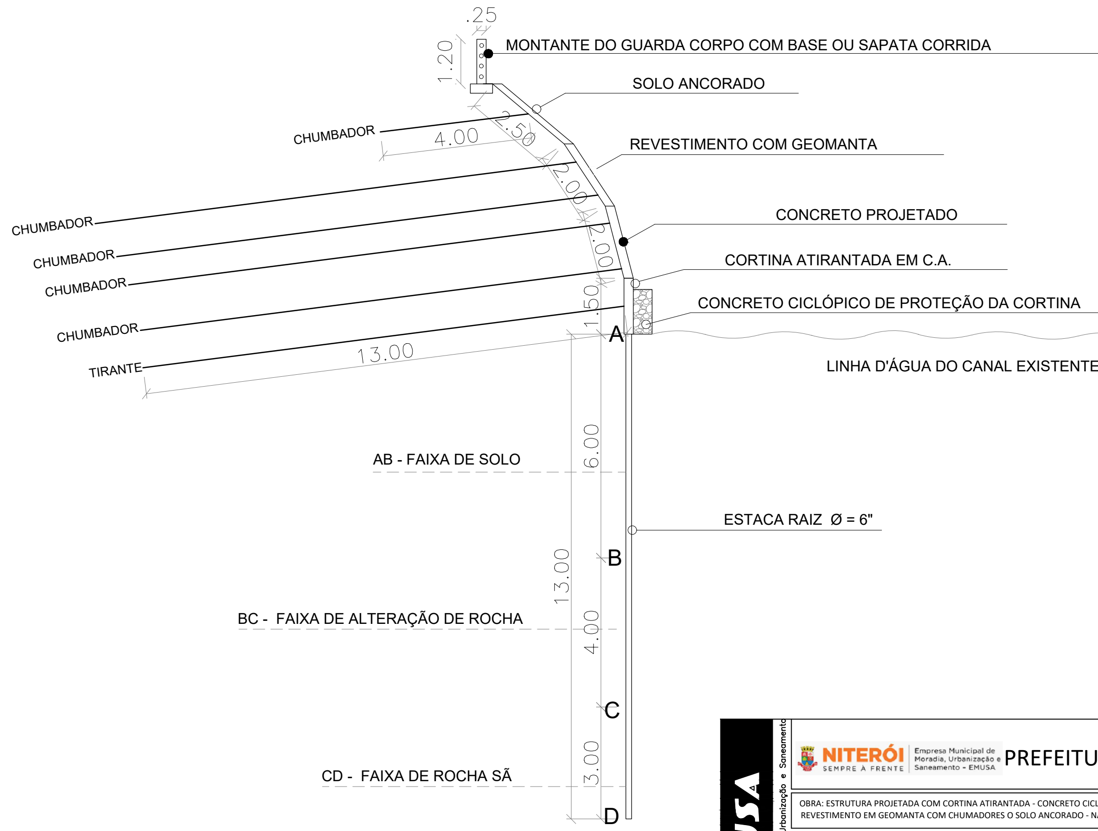
01 CORTE TRANSVERSAL ESC.: 1/100
