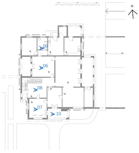
RESIDÊNCIA - TÉRREO
