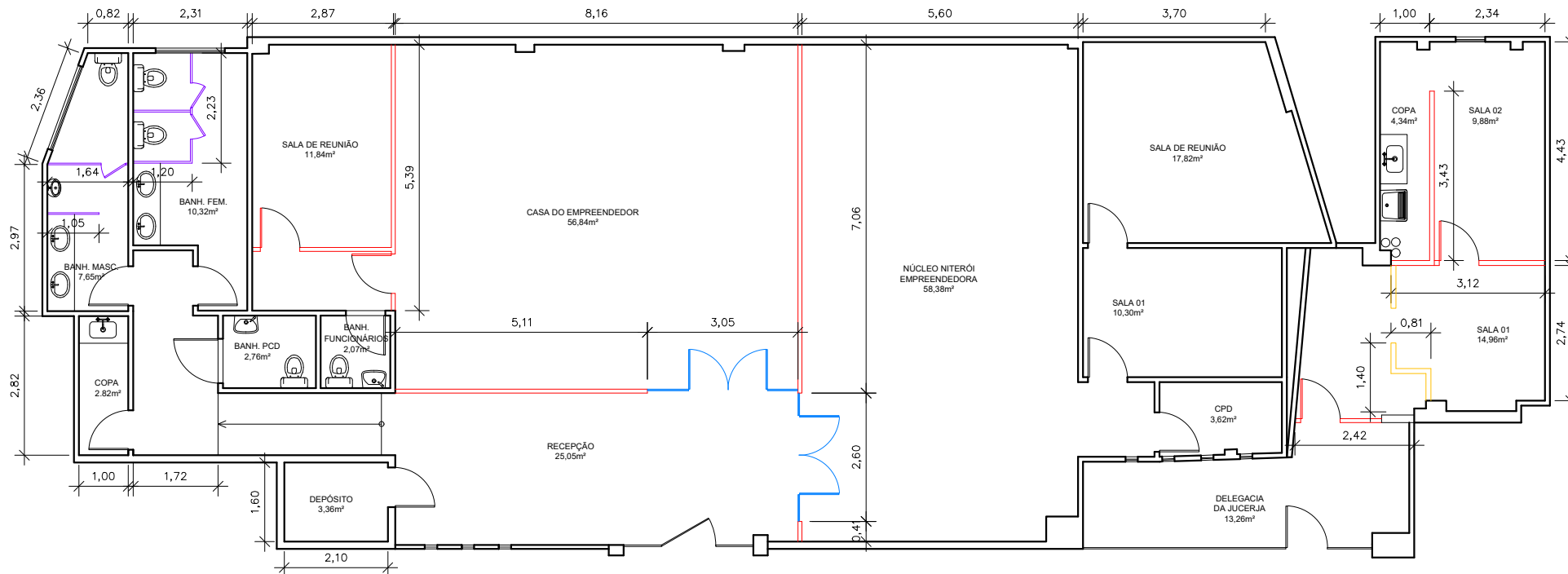
03 PLANTA BAIXA ESCALA 1:125
