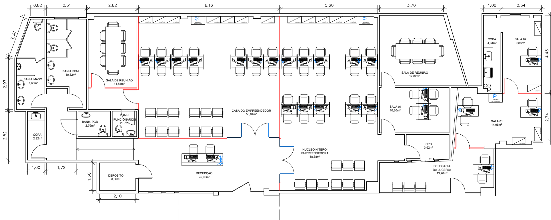
02 PLANTA BAIXA ESCALA 1:125
