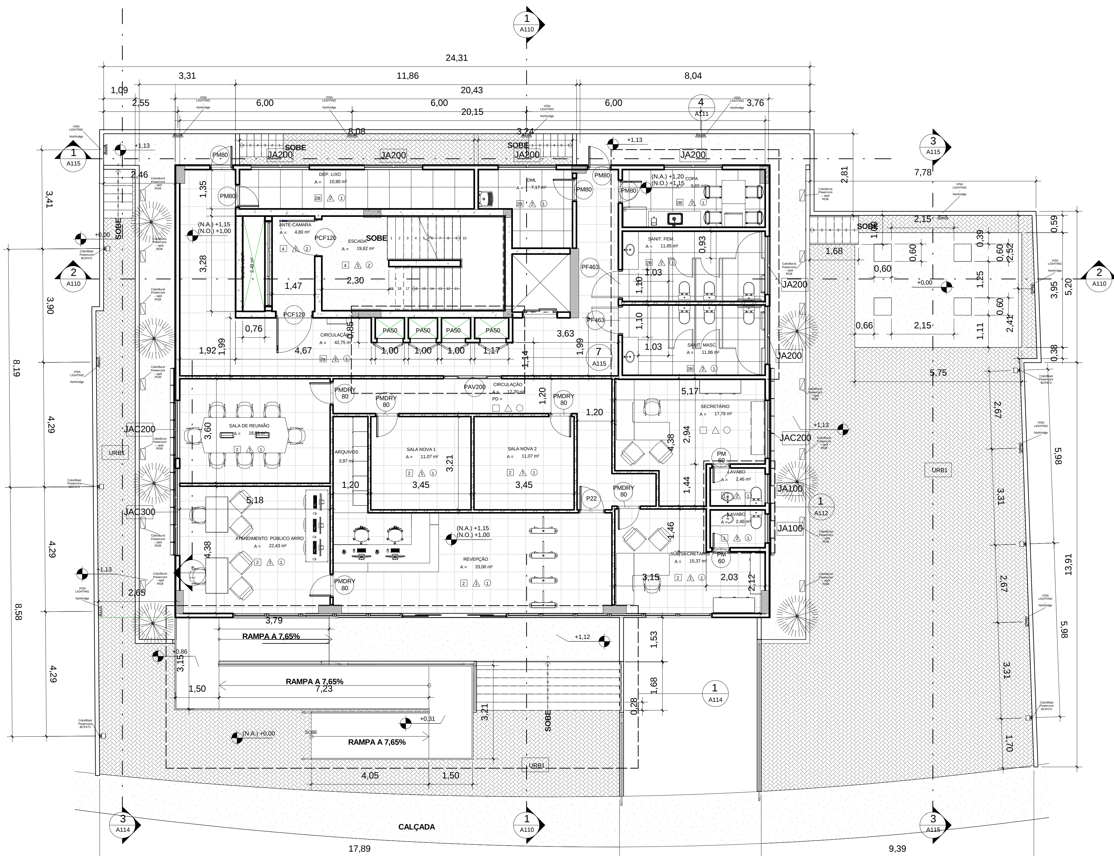
1 NV TÉRREO 1:75
