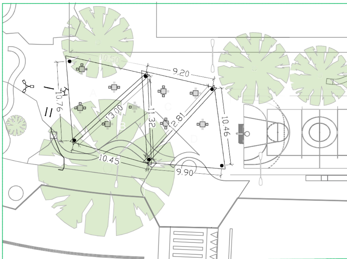
01 AFASTAMENTO ENTRE OS POSTES ONDE SERÃO FIXADAS AS COBERTURAS esc 1:250
