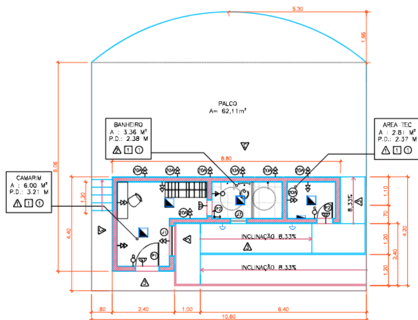
01 PLANTA BAIXA - CAMARIM E PALCO
