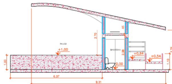
03 CORTE TRANSVERSAL - CAMARIM E PALCO
