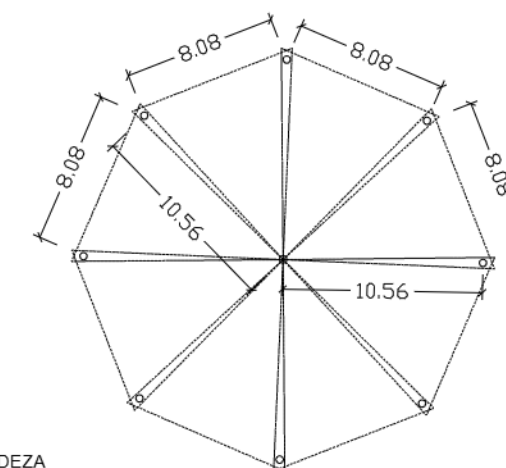
01 AFASTAMENTO ENTRE OS POSTES ONDE SERÃO FIXADAS AS COBERTURAS sem escala
