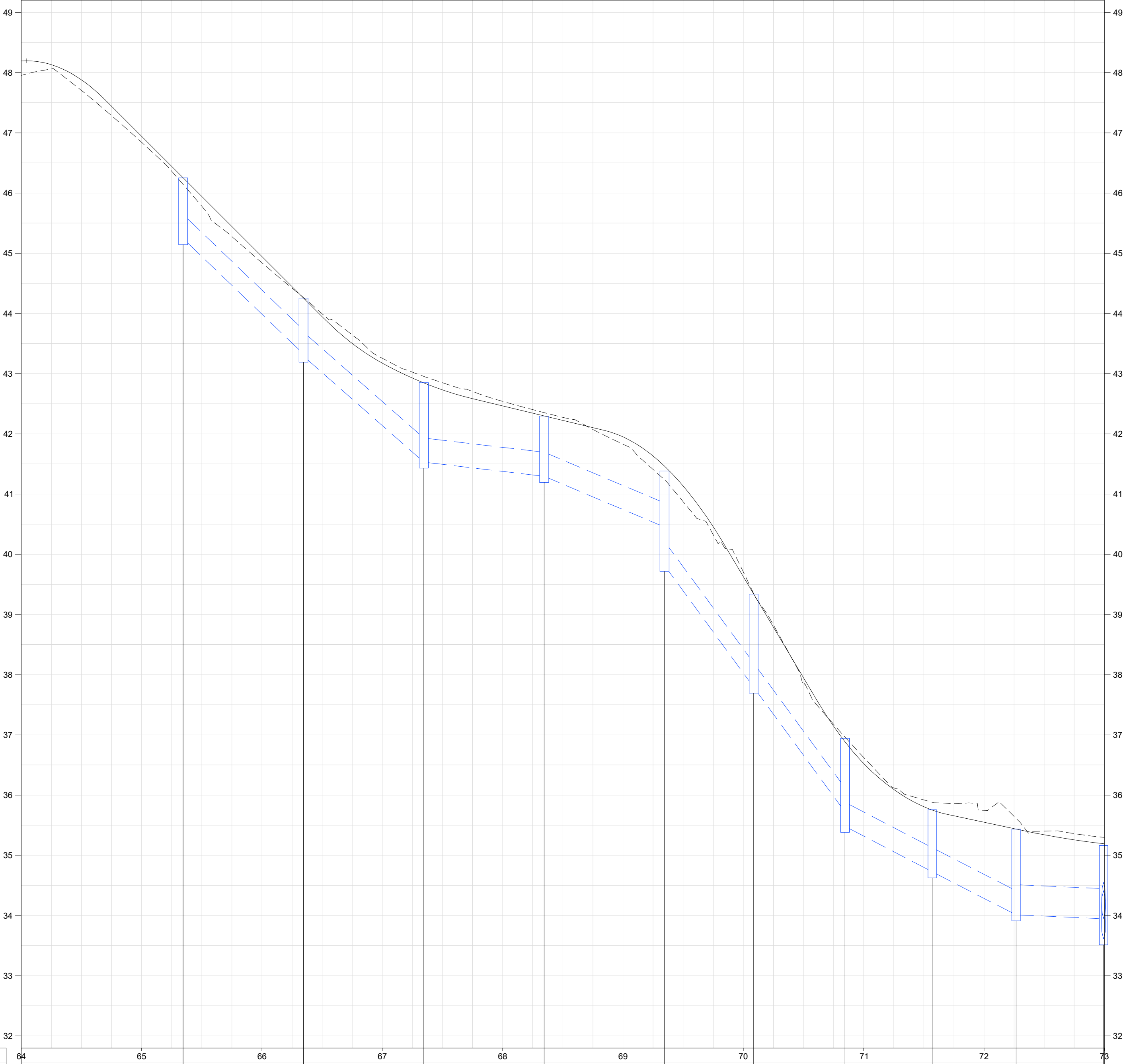
EIXO 50 - RUA DAS AMETISTAS (2-3)
