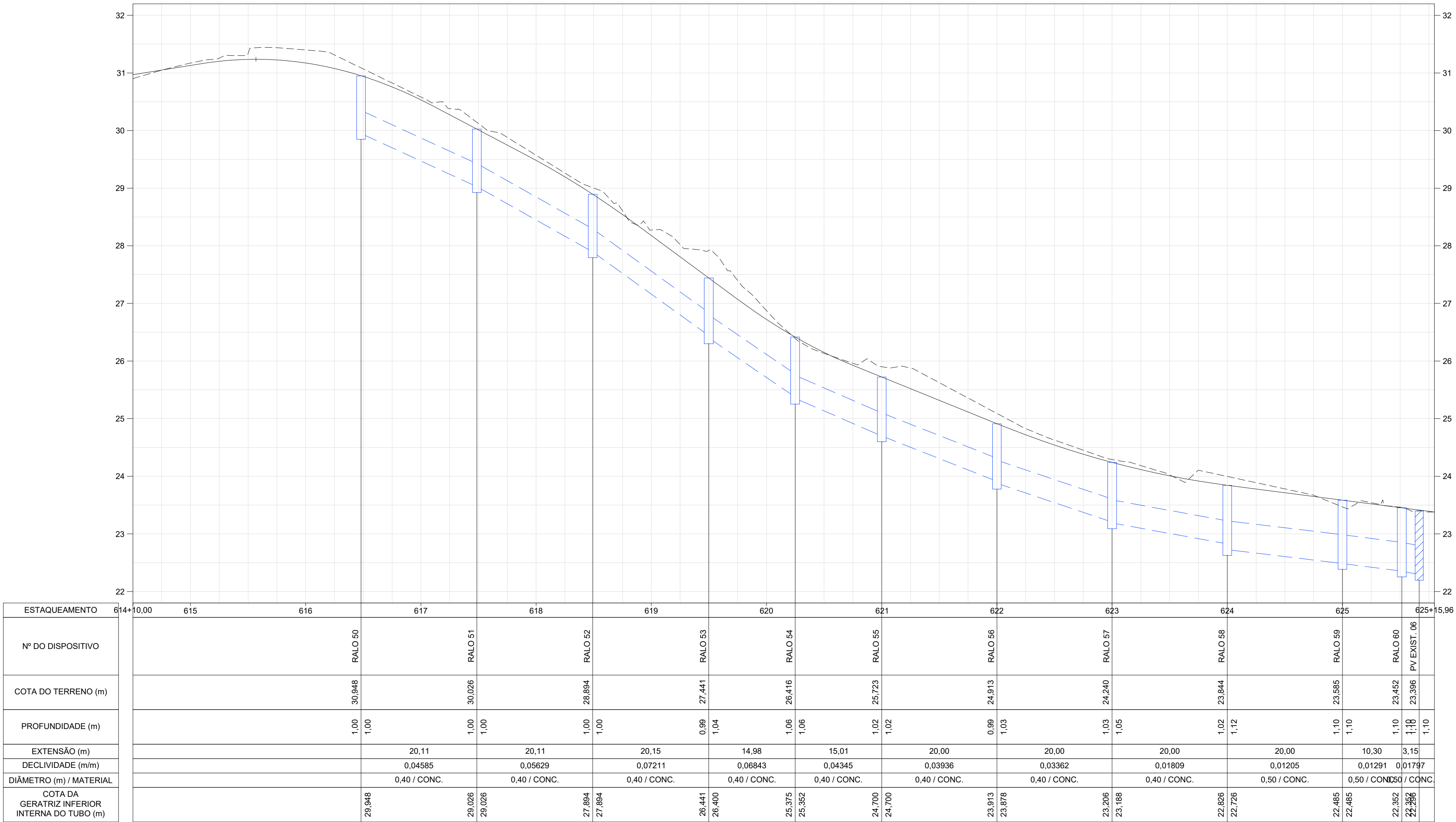
EIXO 600 - RUA DOS CRISTAIS (2-2)
