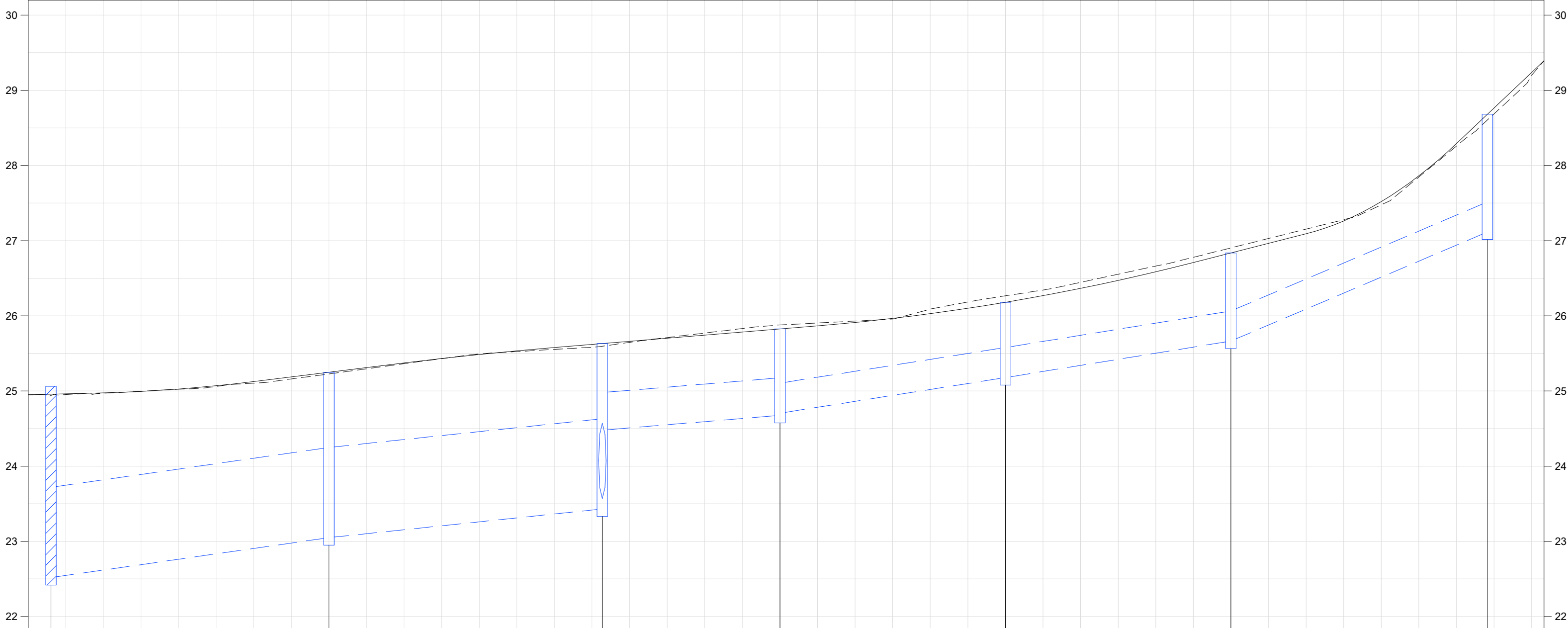
PERFIL - EIXO 300 - RUA LUIZ FERNANDO MARTINS
