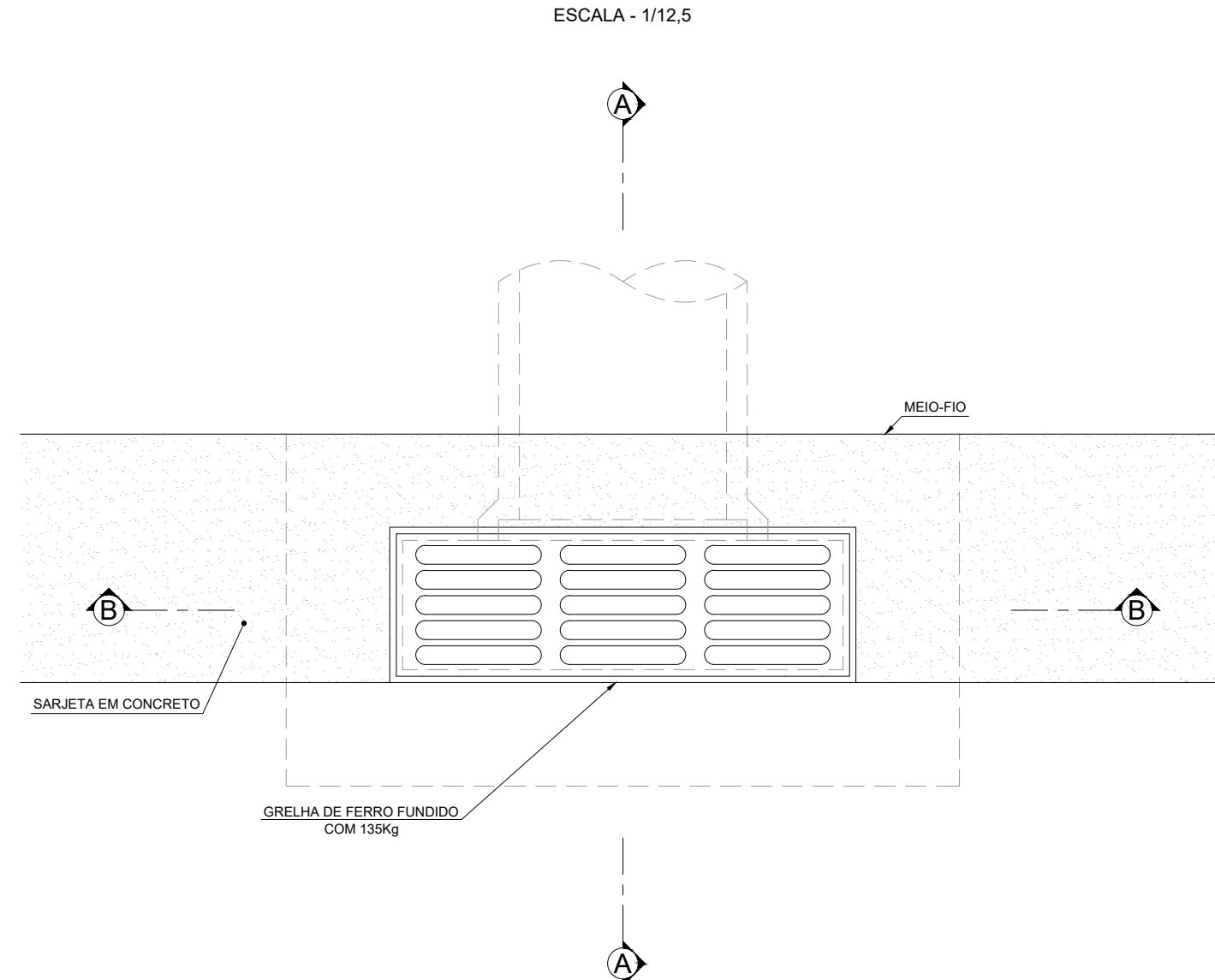
CORTE AA ESCALA - 1/12.5
