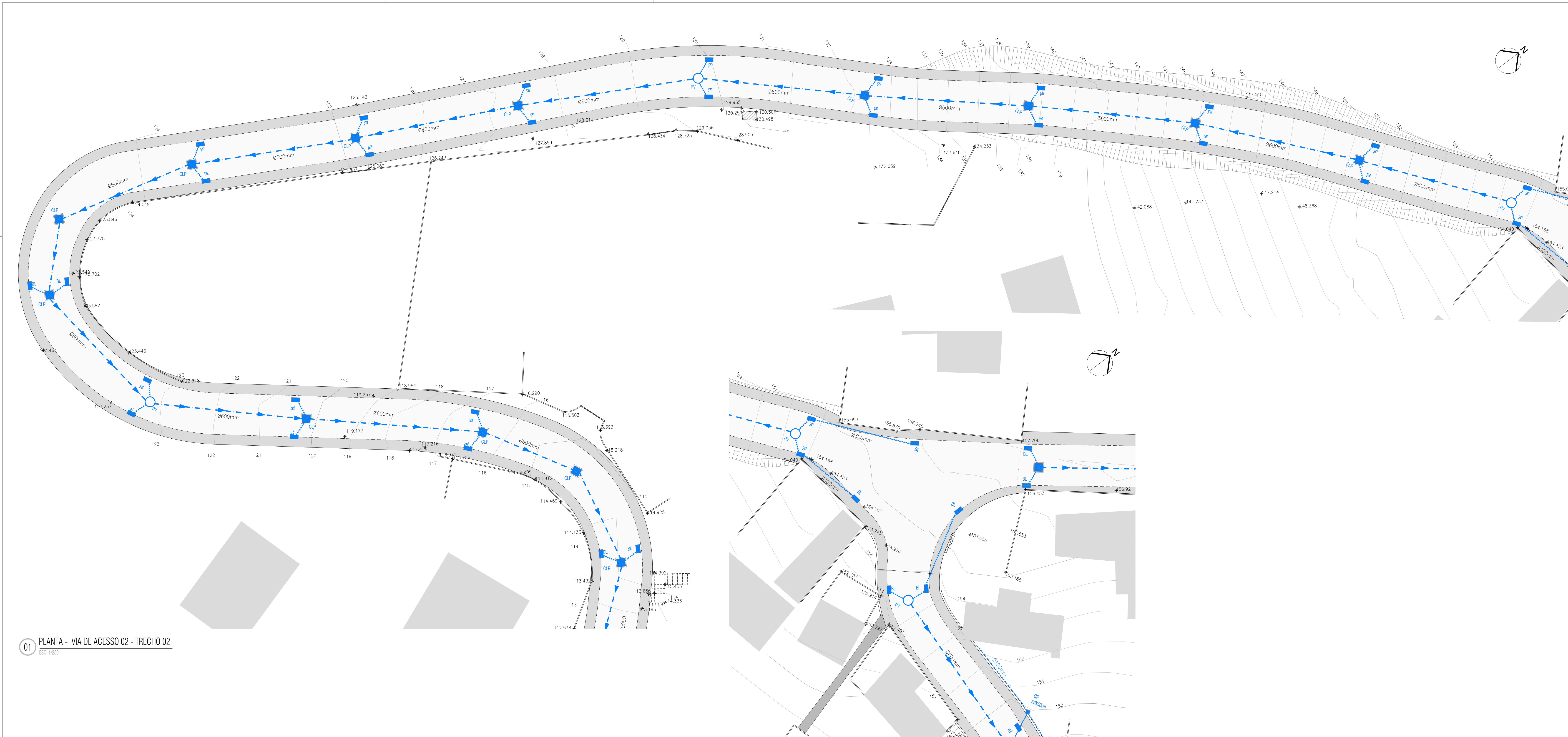
04 PLANTA - VIA DE ACESSO 02 - TRECHO 03 ESC. 1:100
