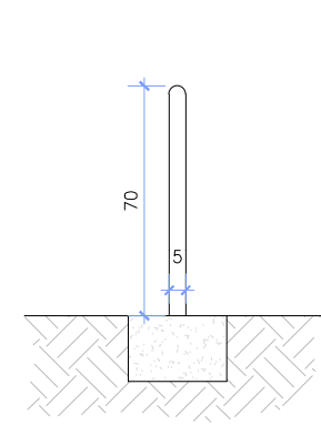
06 PARA-CICLO — VISTA FRONTAL ESC. 1/5
