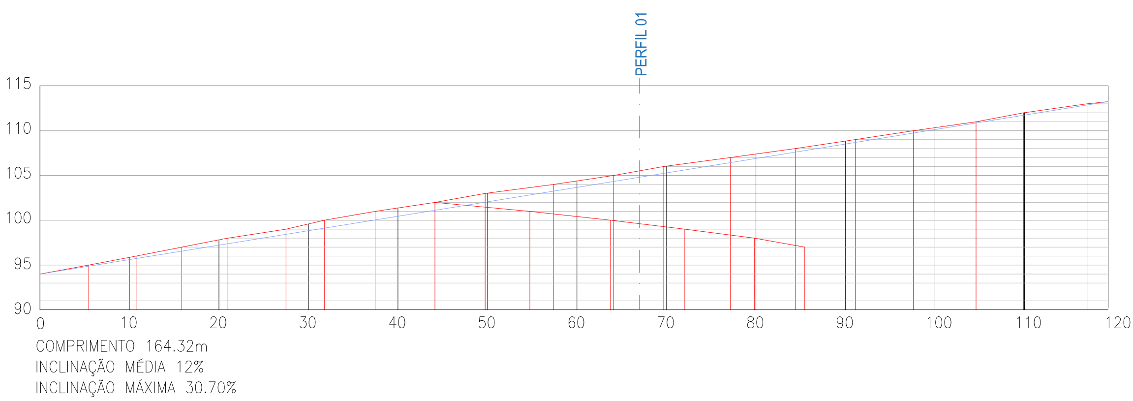
02 PERFIL LONGITUDINAL - VIA 01 (TRECHO 01 E 02) ESC. 1/500
