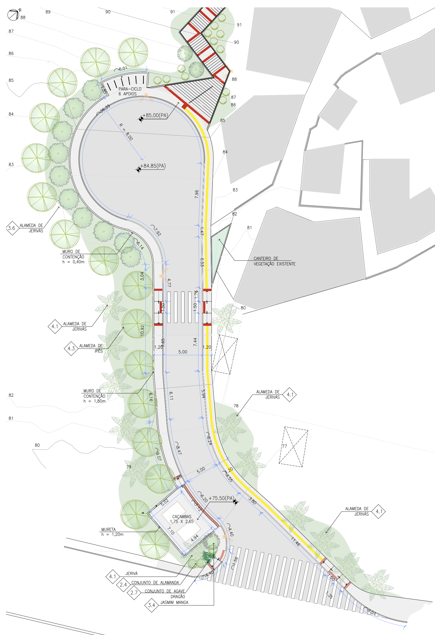
02 ACESSO 01 - PLANTA DE PISO E PAISAGISMO ESC. 1/200
