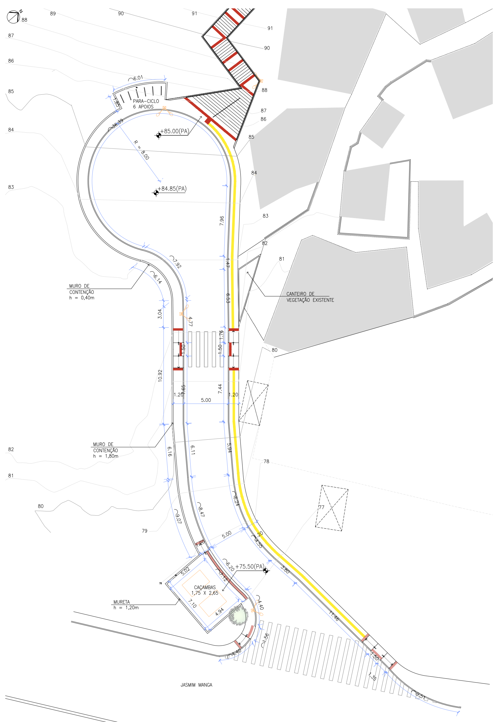
03 ACESSO 01 - PLANTA DE ACESSIBILIDADE ESC. 1/200
