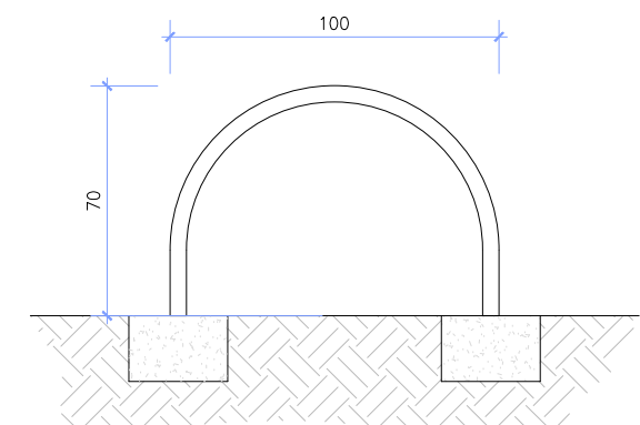
07 PARA-CICLO — VISTA LATERAL ESC. 1/5
