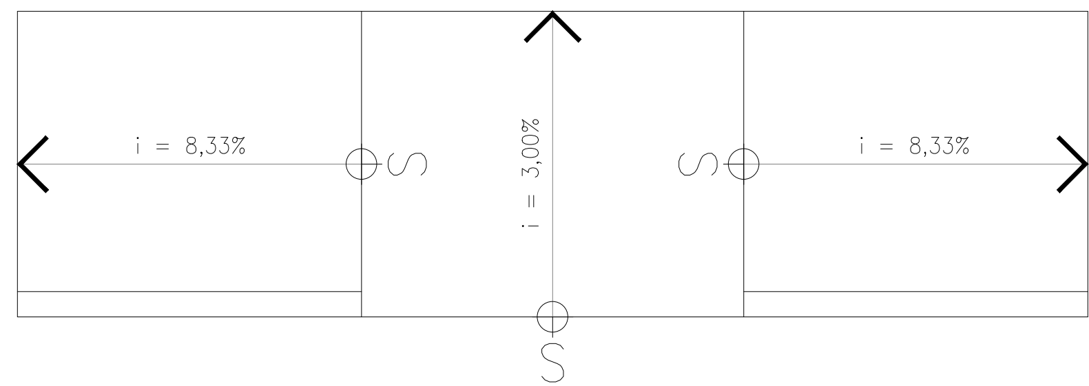
05 PASSEIO REBAIXADO - NBR 9050 ESC. 1/20
