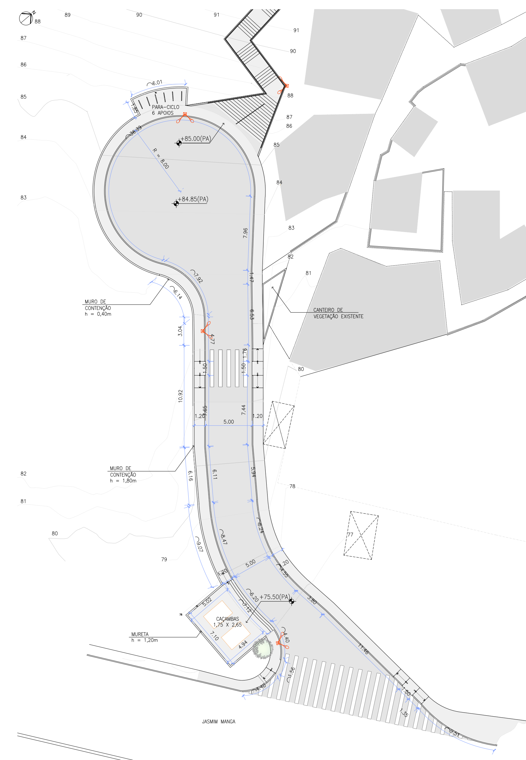
04 ACESSO 01 - PLANTA DE ILUMINAÇÃO ESC. 1/200
