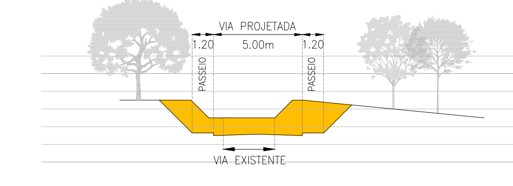
06 PERFIL 04 - VIA DE ACESSO 01 ESC: 1/250
