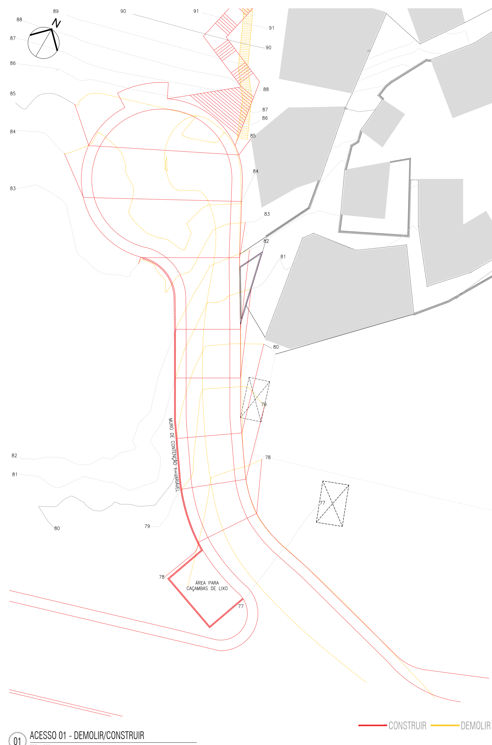
01 ACESSO 01 - DEMOLIR/CONSTRUIR ESC. 1/200
