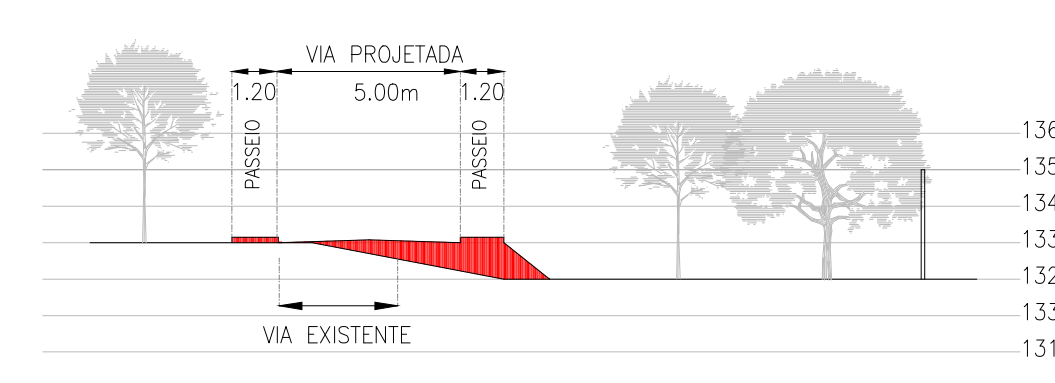
05 PERFIL 03 - VIA DE ACESSO 01 ESC: 1/250
