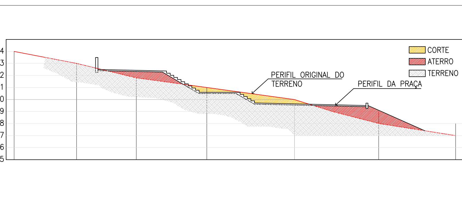
06 PERFIL TRANSVERSAL ESC. 1/250
