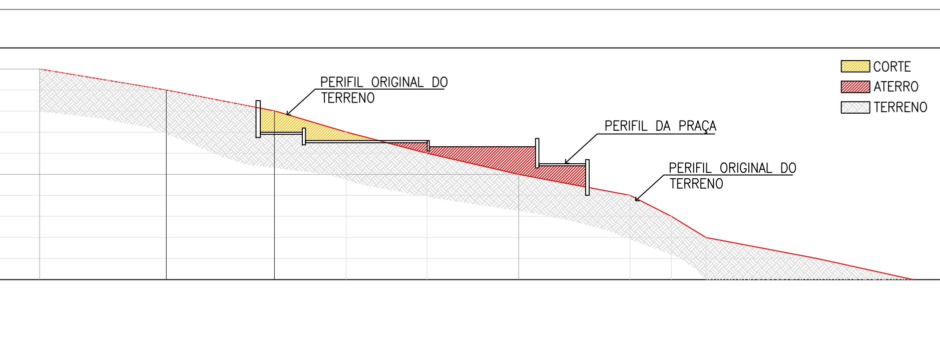
07 PERFIL TRANSVERSAL ESC. 1/250
