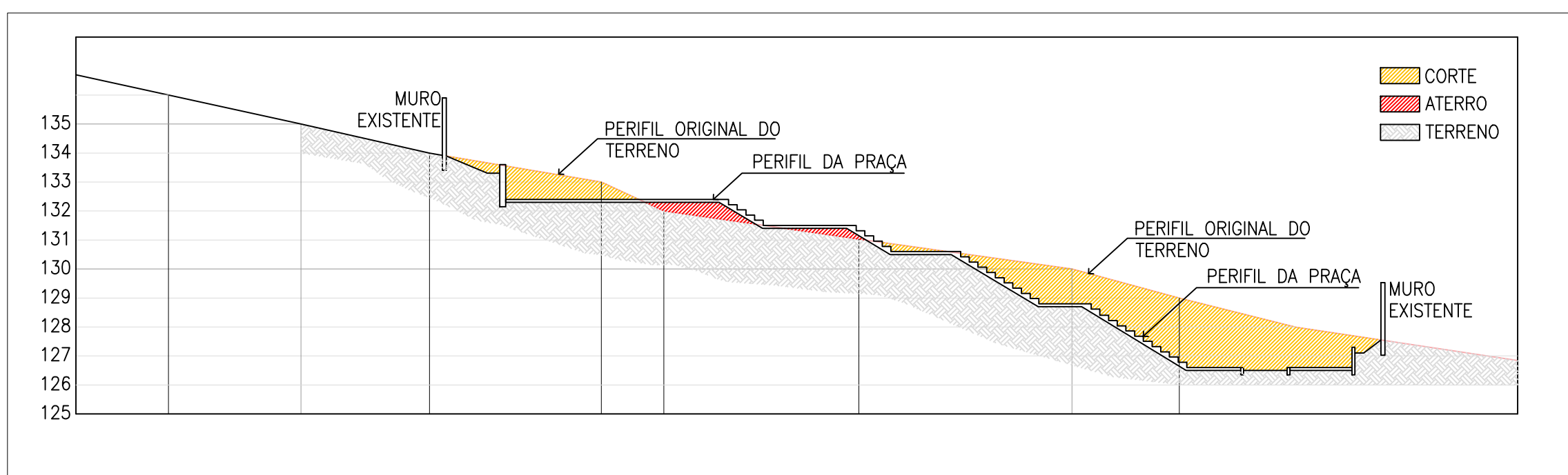
04 PERFIL TRANSVERSAL ESC. 1/250
