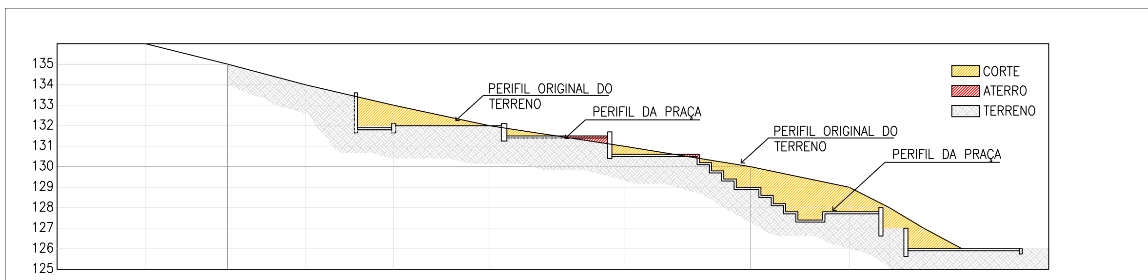
03 PERFIL TRANSVERSAL ESC. 1/250
