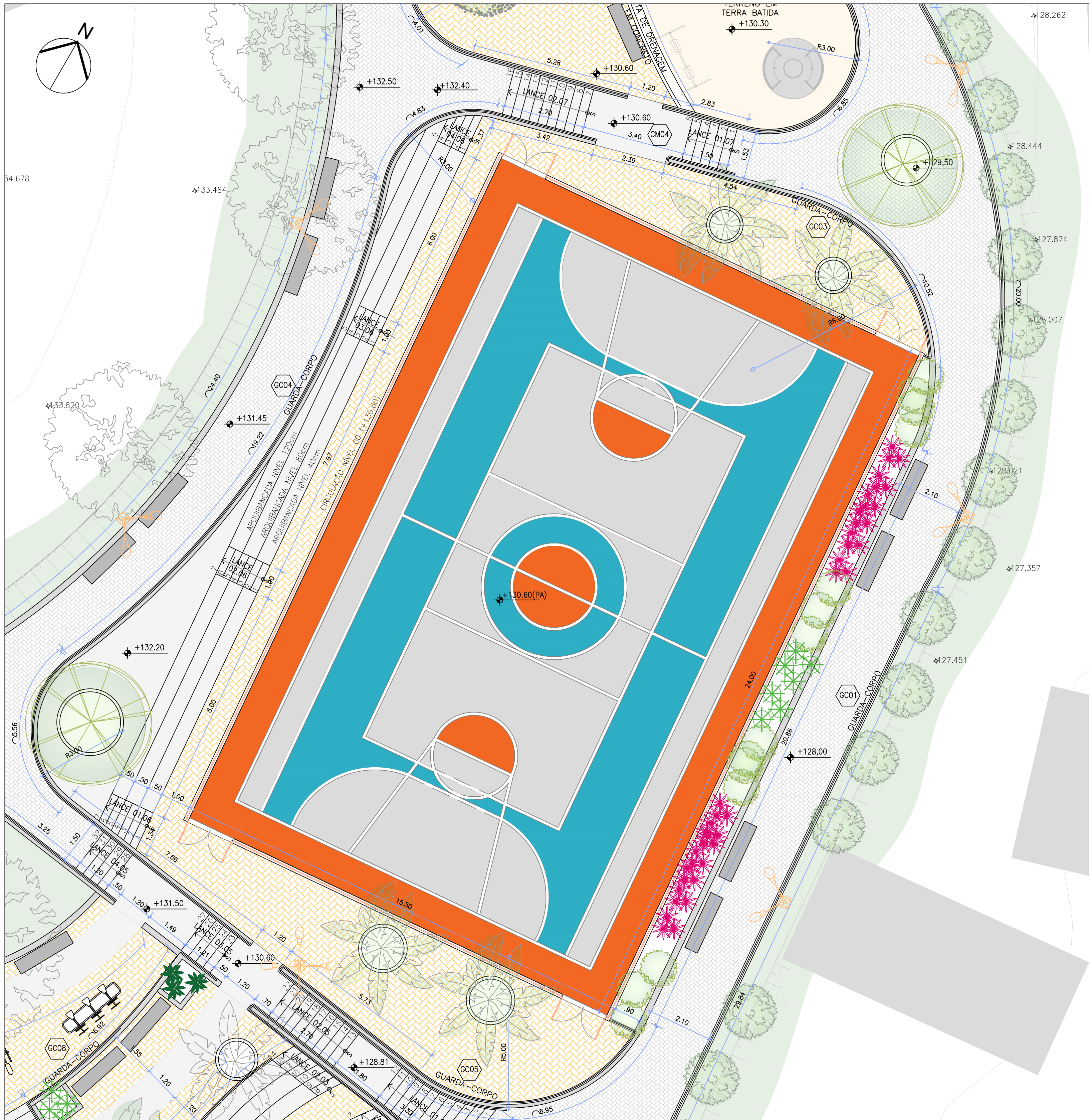
01 PLANTA - ÁREA DE LAZER - TRECHO 2 - QUADRA RECREATIVA
