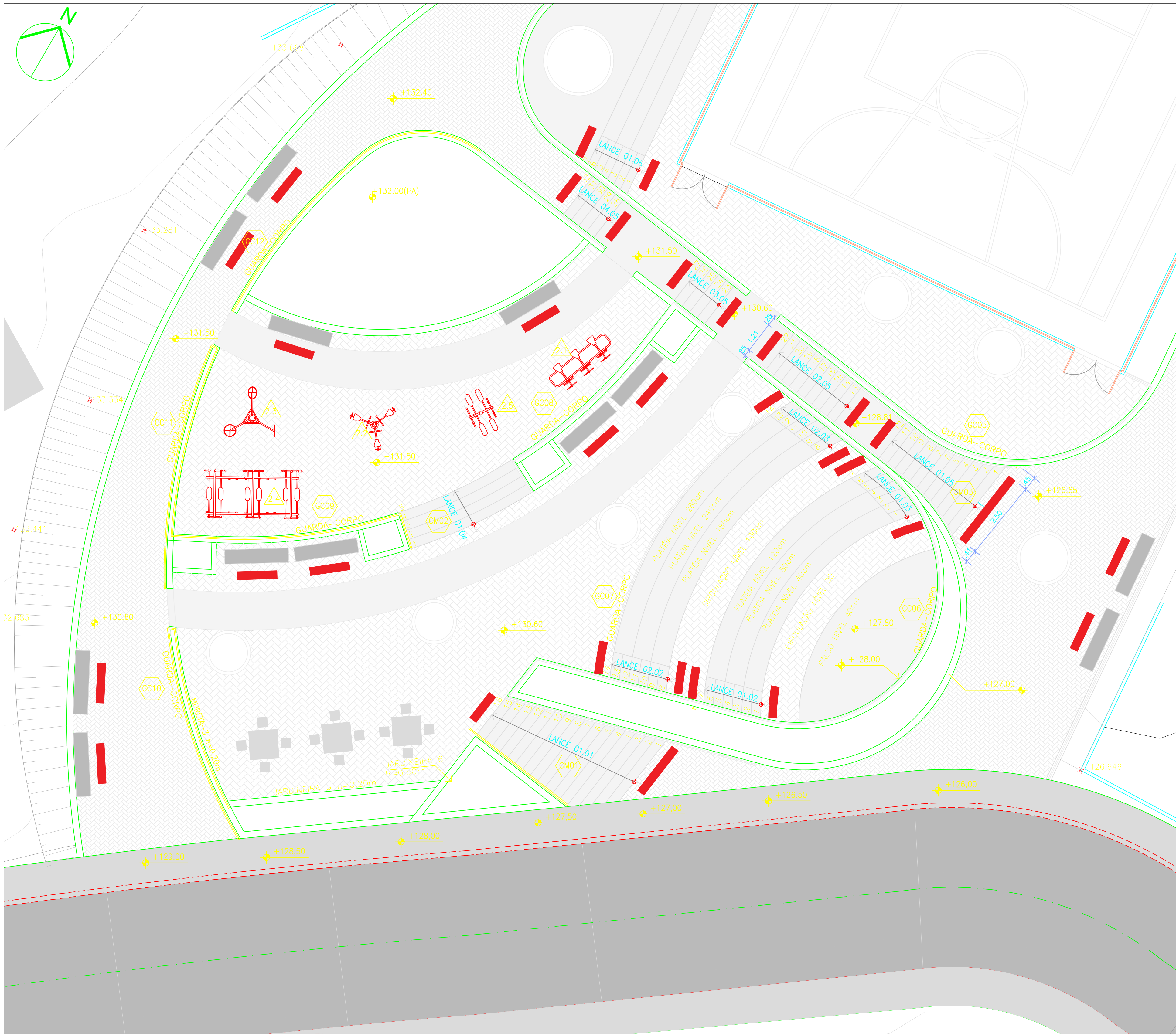
01 ACESSIBILIDADE-ÁREA DE LAZER - TRECHO 3 ESC: 1/100
