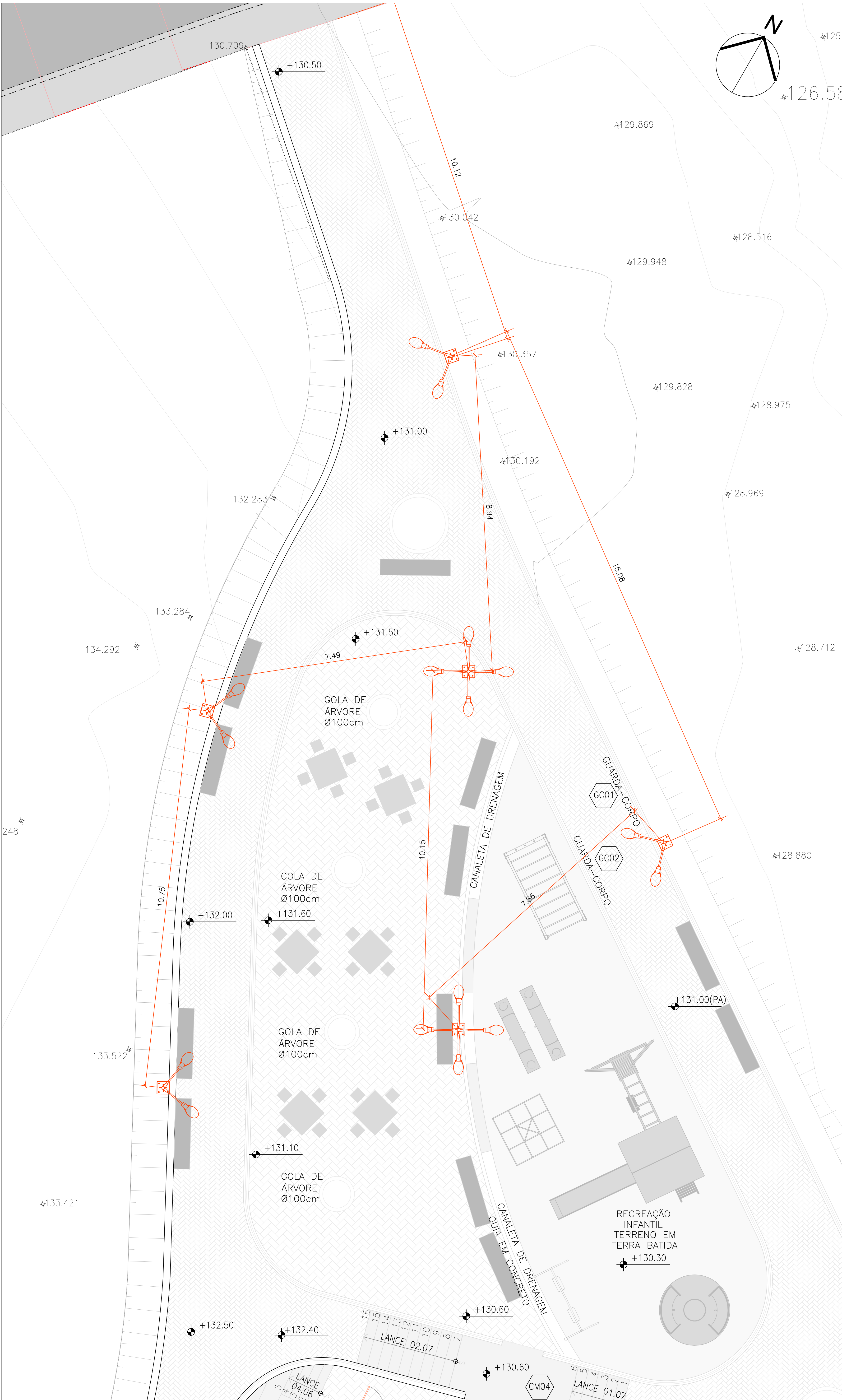
01 ILUMINAÇÃO - ÁREA DE LAZER - TRECHO 1 - RECREAÇÃO INFANTIL ESC: 1/100
