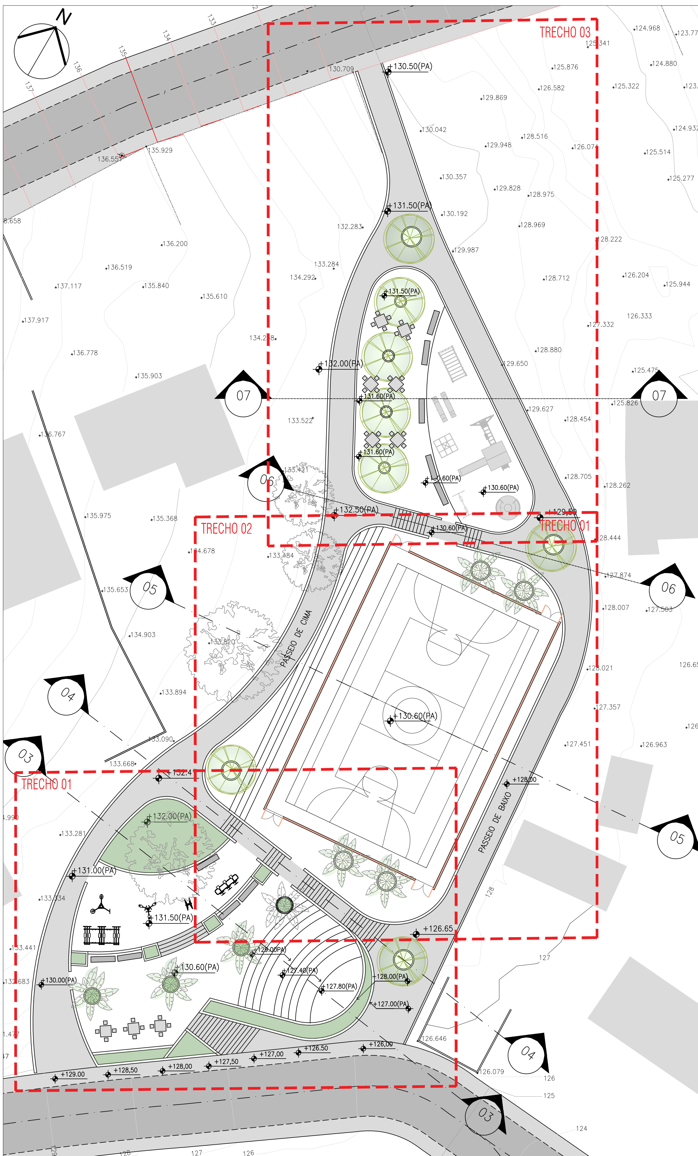
01 ÁREA DE LAZER - IMPLANTAÇÃO GERAL ESC. 1/250
