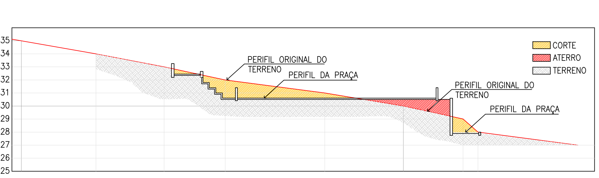
05 PERFIL TRANSVERSAL ESC. 1/250
