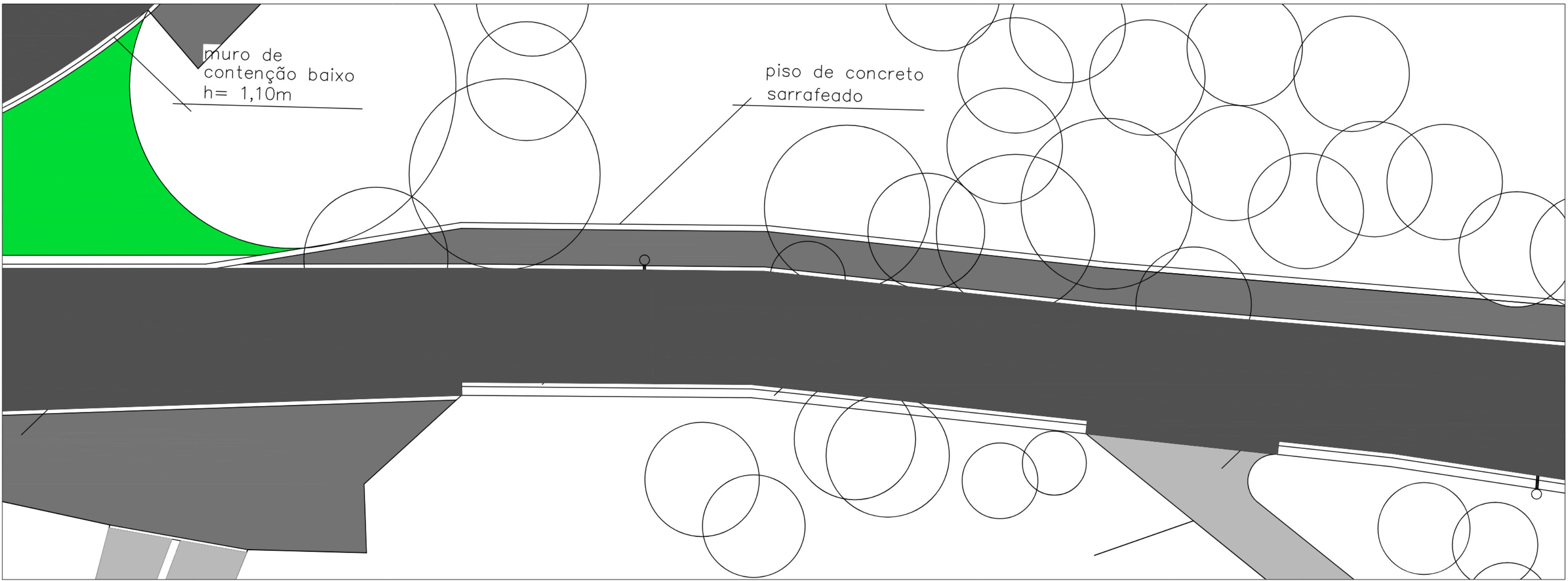
1 DETALHE ESQUEMÁTICO 3 Esc. 1/100
