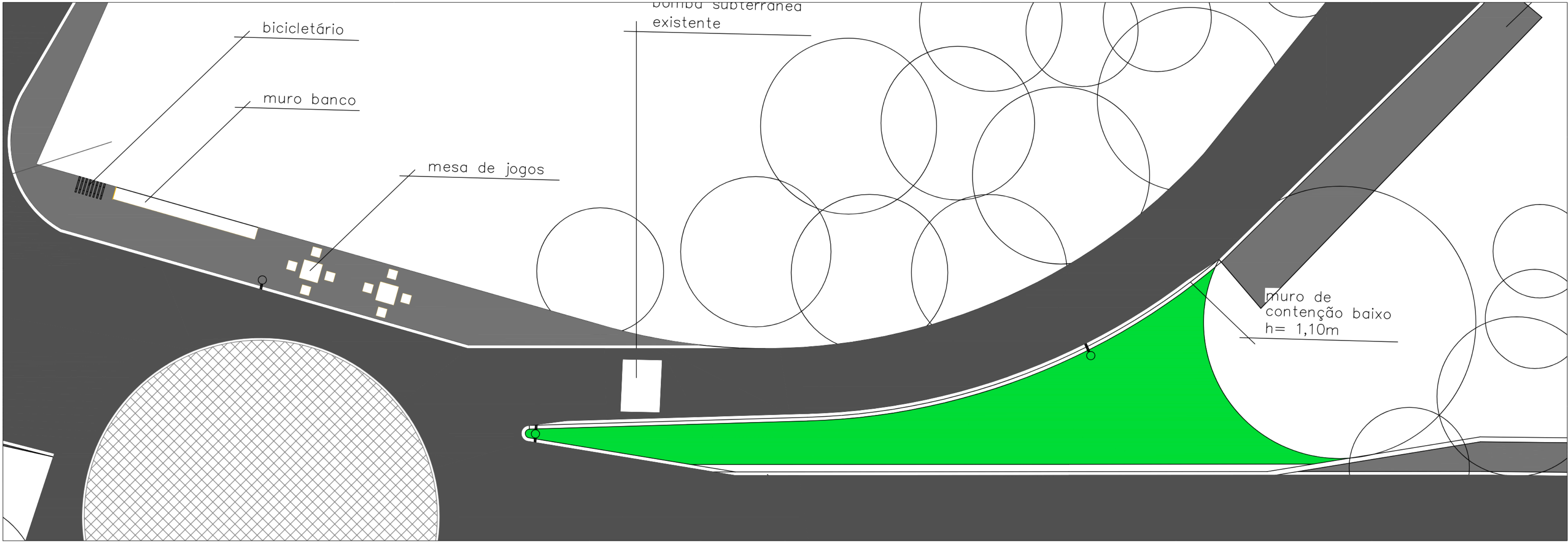
2 DETALHE ESQUEMÁTICO 4 Esc. 1/100
