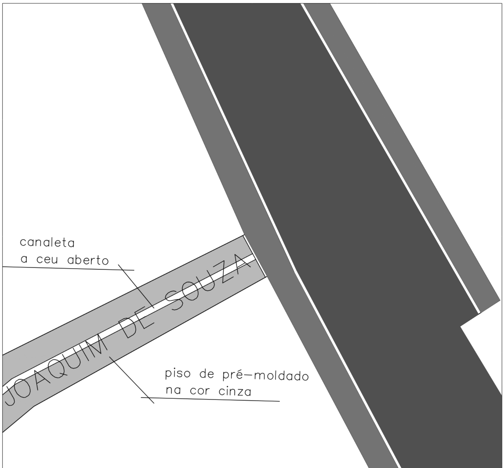
2 DETALHE ESQUEMÁTICO 6 ESC. 1/100
