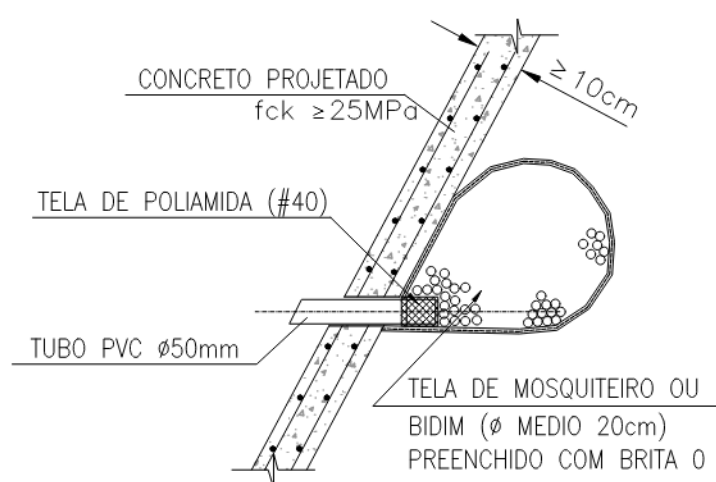
DETALHE 1 (DRENO) S/ESC.
