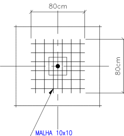
DETALHE 3 (FRETAGEM) S/ESC.
