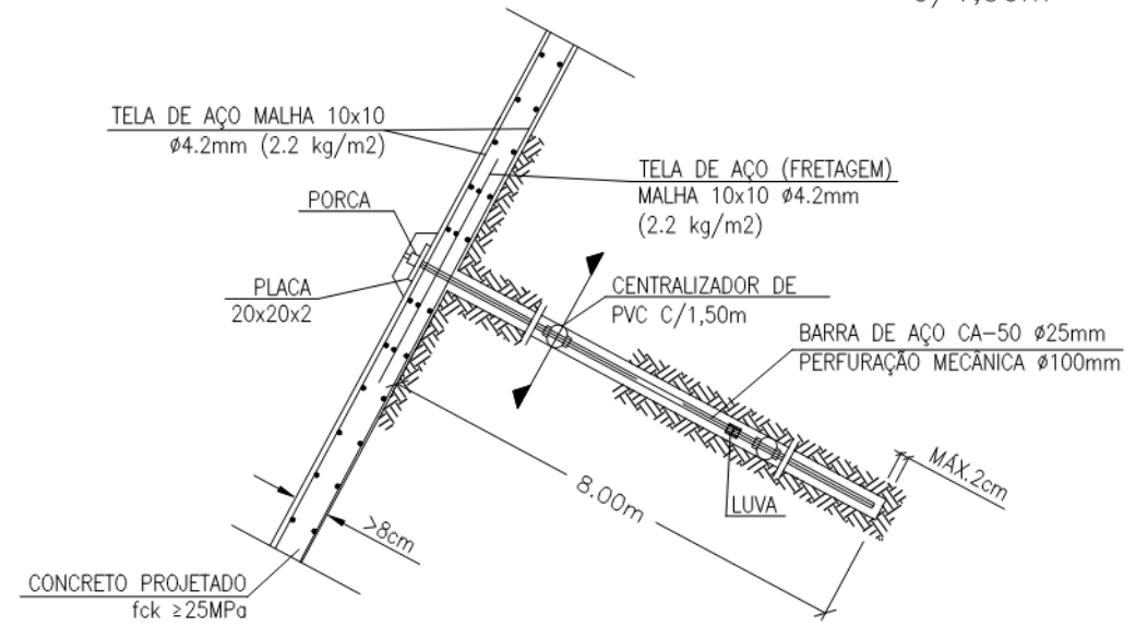
SOLO GRAMPEADO VISTA FRONTAL TÍPICA S/ESC.
