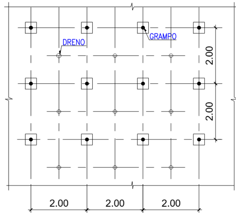
SOLO GRAMPEADO VISTA FRONTAL TÍPICA S/ESC.
