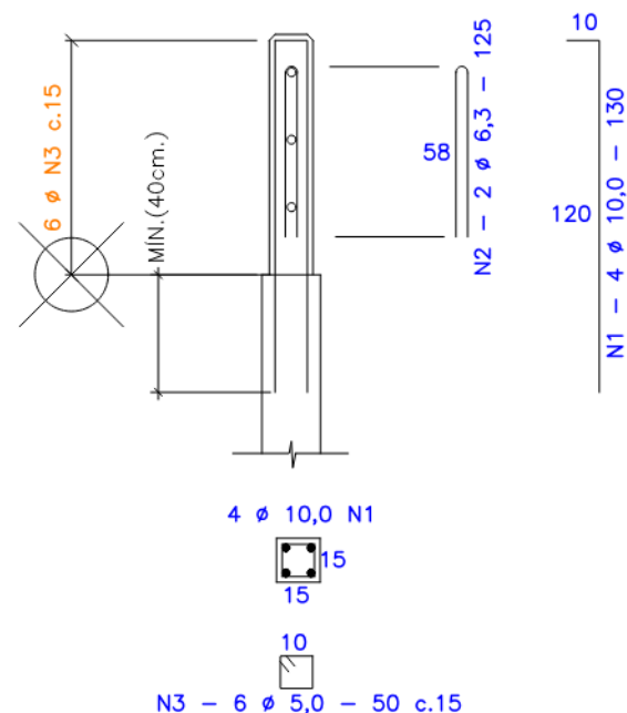
COLONAS - ARMAÇÕES
